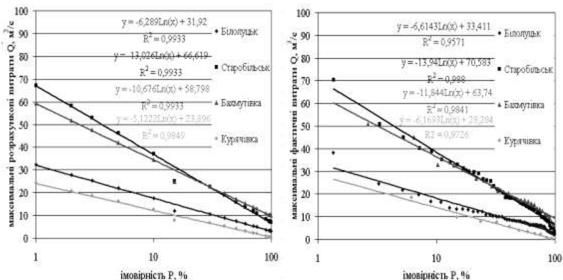
Рис. 1. Максимальні витрати стоку за гідропостами
